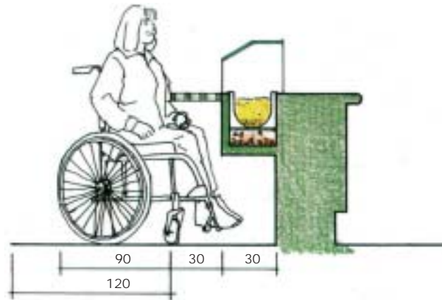
Dimensiones básicas de una barra de autoservicio para la aproximación frontal de una persona en silla de ruedas
